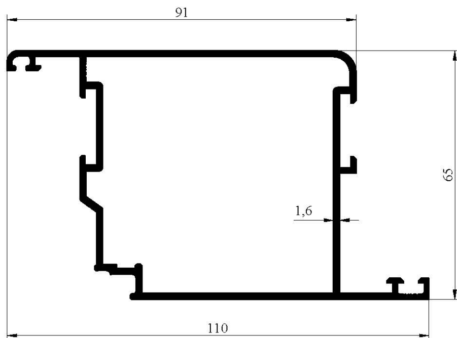
1158 1,482 kg/m
