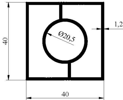
1128 0,772 kg/m
