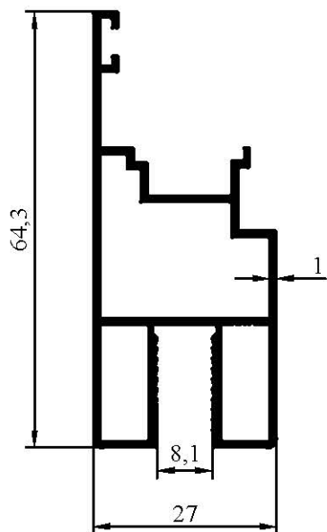
1113 0,618 kg/m
