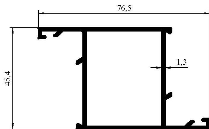
7004 0,828 kg/m
