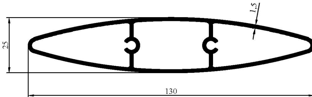
7026 1,323 kg/m
