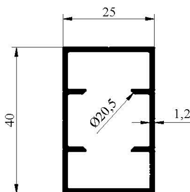
1180 0,463 kg/m
