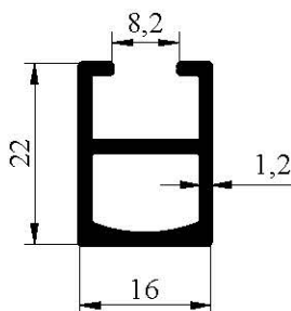
7028 0,265 kg/m
