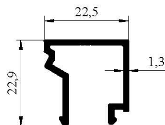
1160 0,260 kg/m
