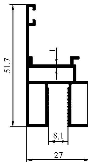
1114 0,528 kg/m
