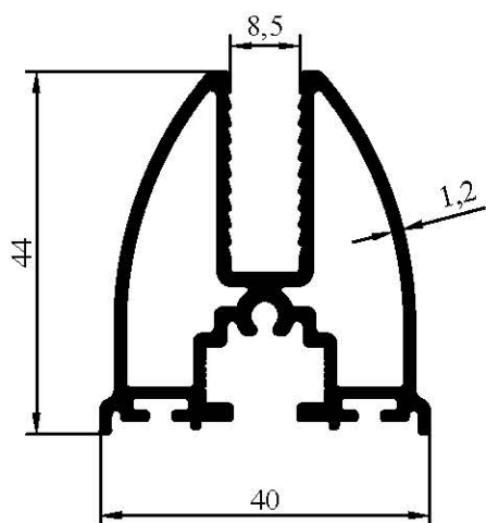
1148 0,864 kg/m
