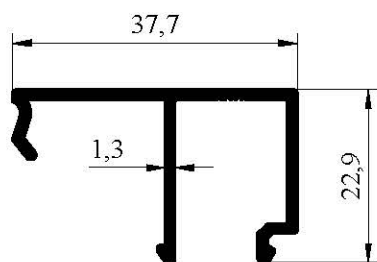
1159 0,333 kg/m
