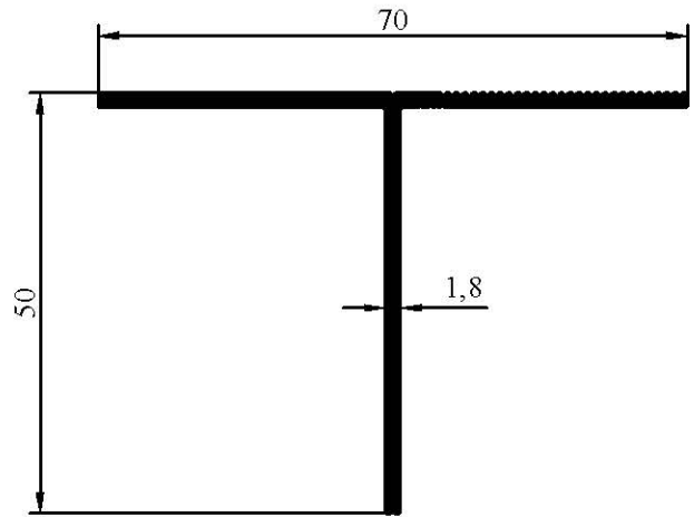
1082 0,547 kg/m
