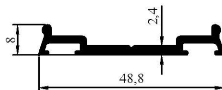
7060 0,353 kg/m
