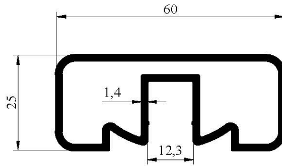
7033 0,768 kg/m
