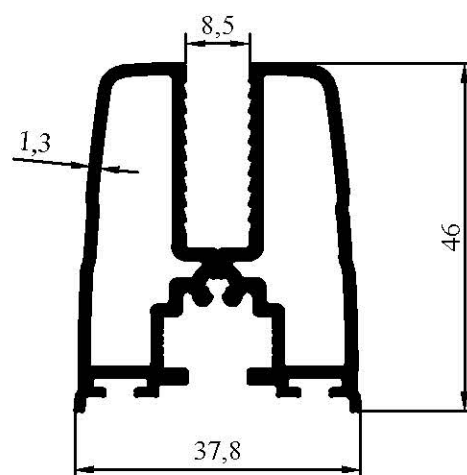
1142 0,957 kg/m
