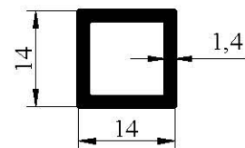
7035 0,191 kg/m
