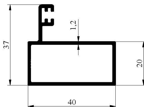
1181 0,485 kg/m
