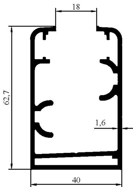
1109 1,209 kg/m
