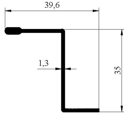
1130 0,279 kg/m
