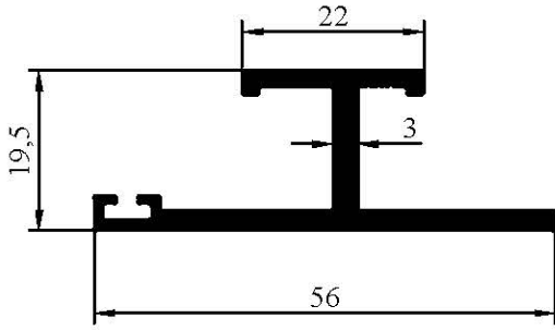
1079 0,629 kg/m
