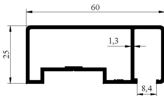
1177 0,678 kg/m
