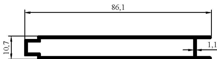
7008 0,563 kg/m
