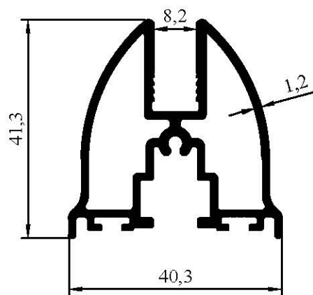
1111 0,778 kg/m
