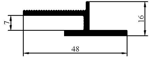
1080 0,444 kg/m
