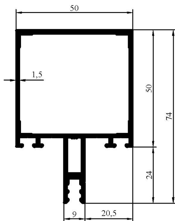
7050 1,184 kg/m
