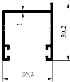
1132 0,257 kg/m
