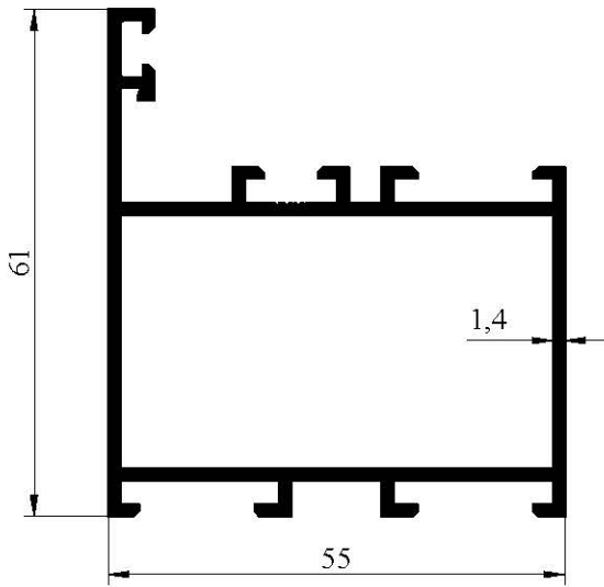
1155 0,976 kg/m
