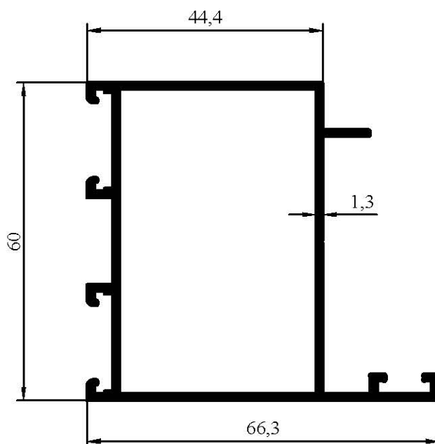
7014 0,946 kg/m
