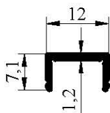
7029 0,064 kg/m
