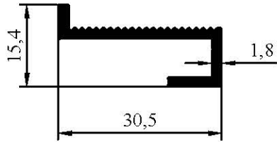
1081 0,252 kg/m
