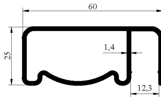
7031 0,678 kg/m
