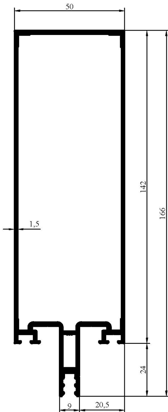
7054 2,065 kg/m
