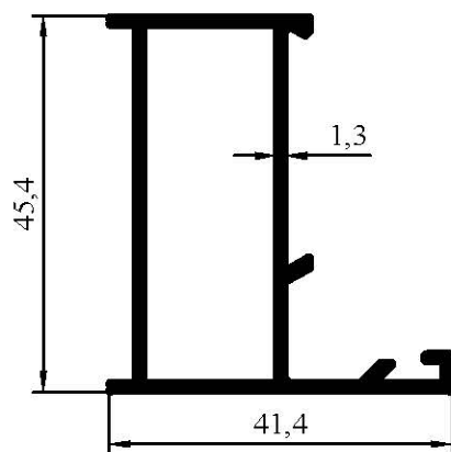
7012 0,587 kg/m
