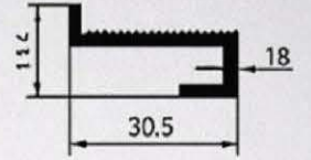
1081 0,252 kg/m
