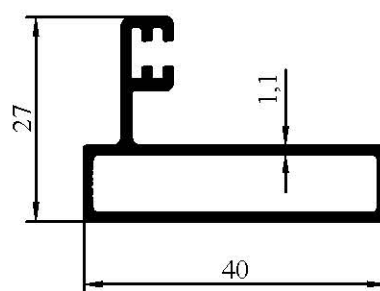
1112 0,398 kg/m
