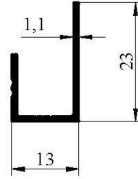
1172 0,136 kg/m
