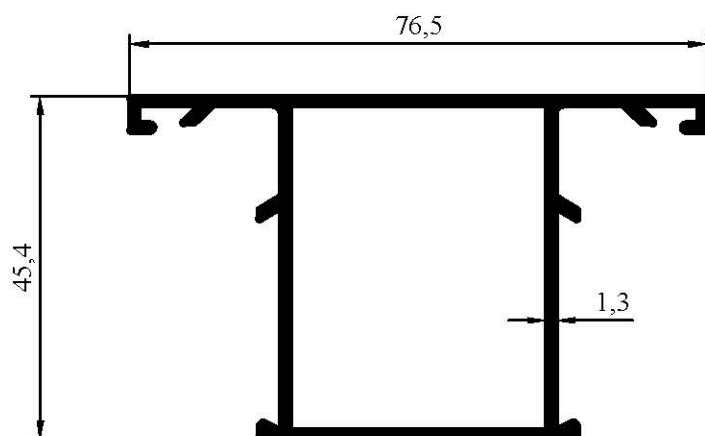
7003 0,828 kg/m
