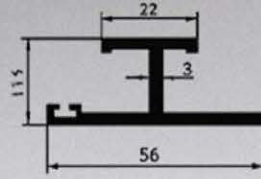
1079 0,629 kg/m
