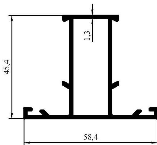
7009 0,700 kg/m
