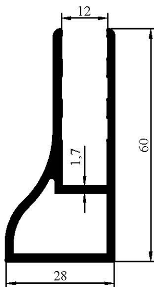
7036 0,792 kg/m
