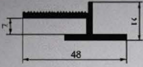
1080 0,444 kg/m
