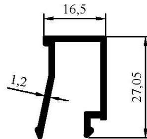
7023 0,244 kg/m
