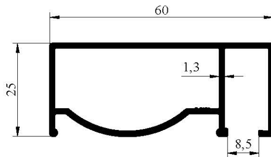
1178 0,648 kg/m
