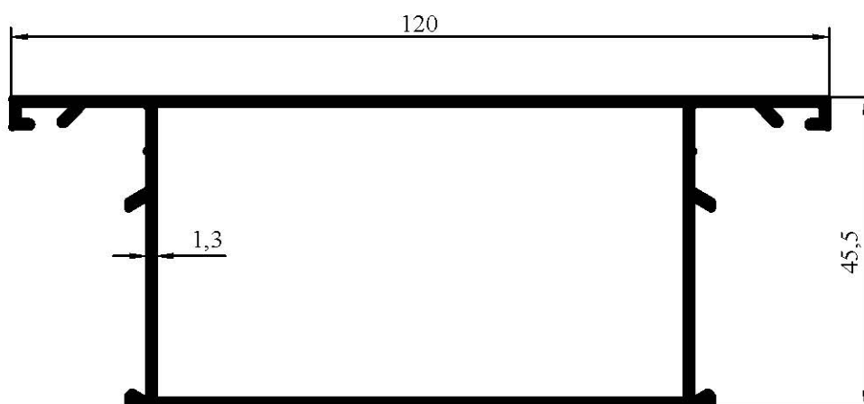
7005 1,130 kg/m
