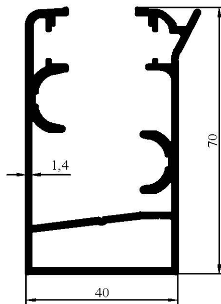
1143 1,276 kg/m
