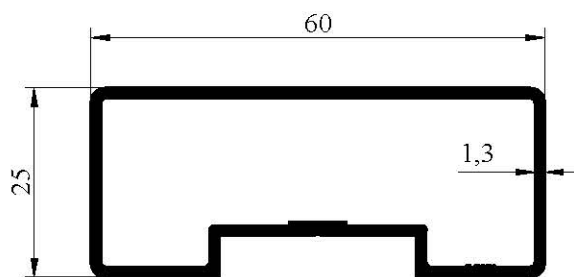
1182 0,623 kg/m
