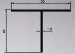
1082 0,547 kg/m
