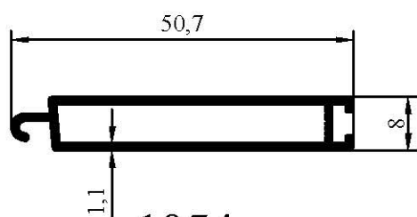
1054 0,333 kg/m
