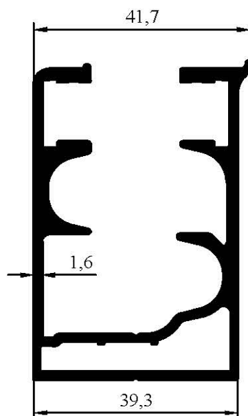
7074 1,252 kg/m
