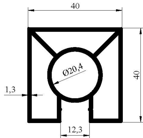
7027 0,914 kg/m
