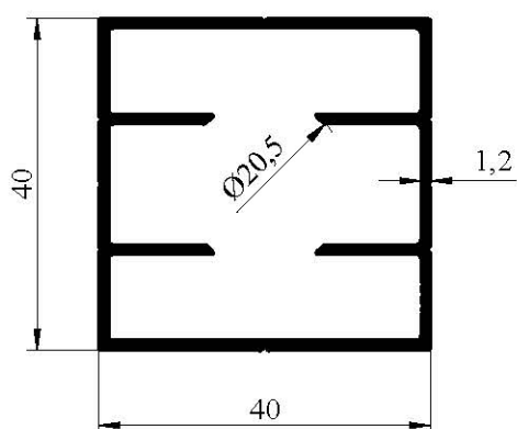
1179 0,659 kg/m
