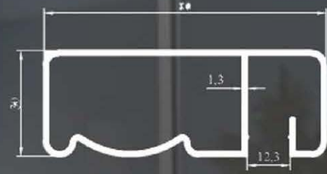
7032 0,830 kg/m
