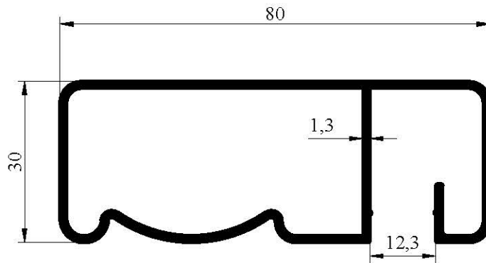
7032 0,830 kg/m
