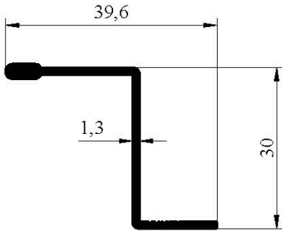
1129 0,260 kg/m
