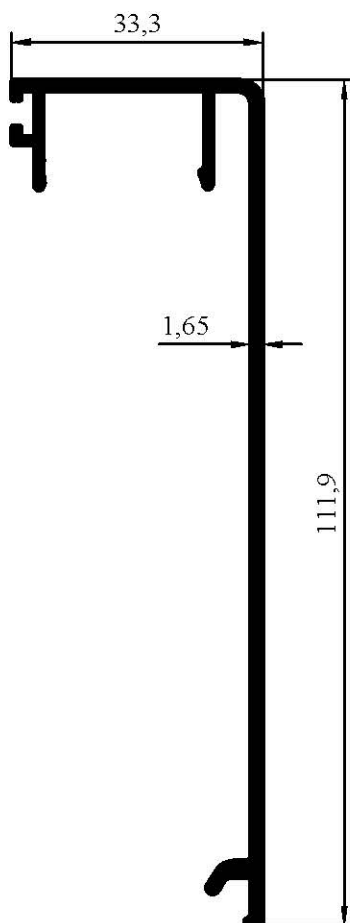
7069 0,763 kg/m
