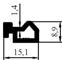
7059 0,172 kg/m
