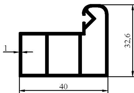
7078 0,496 kg/m
