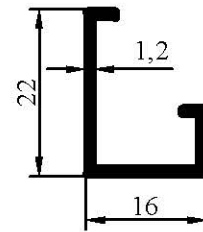
7030 0,162 kg/m
