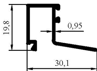
7006 0,201 kg/m
