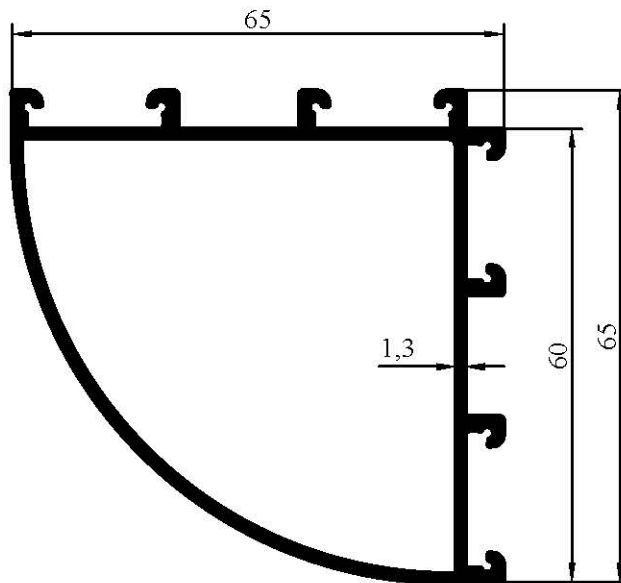
7017 0,997 kg/m
