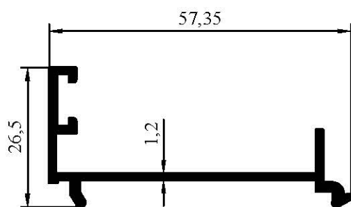
7021 0,366 kg/m
