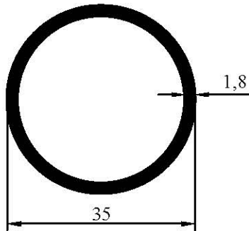
7040 0,509 kg/m
