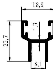
7079 0,222 kg/m
