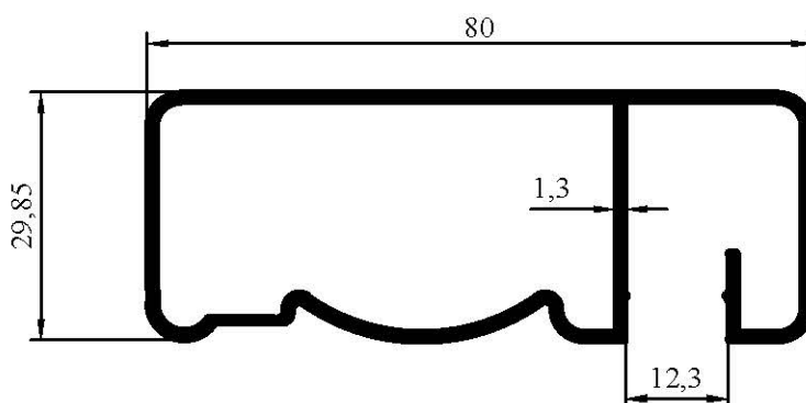
7072 0,827 kg/m
