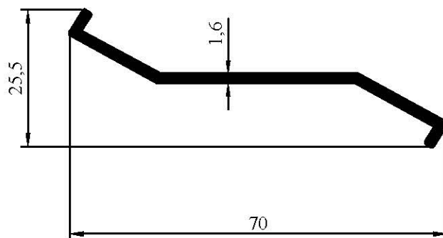
7062 0,353 kg/m
