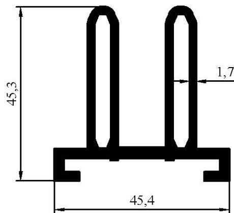
7058 1,178 kg/m
