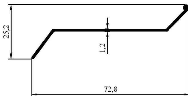
1003 0,282 kg/m
