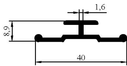
7067 0,237 kg/m
