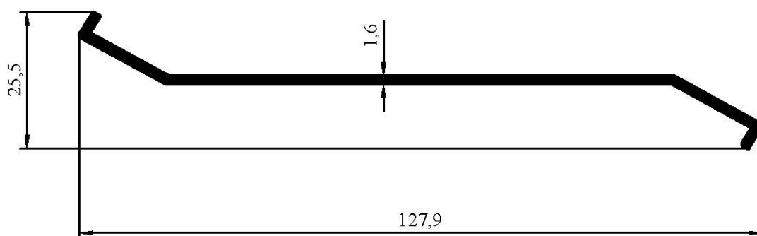
7061 0,604 kg/m
