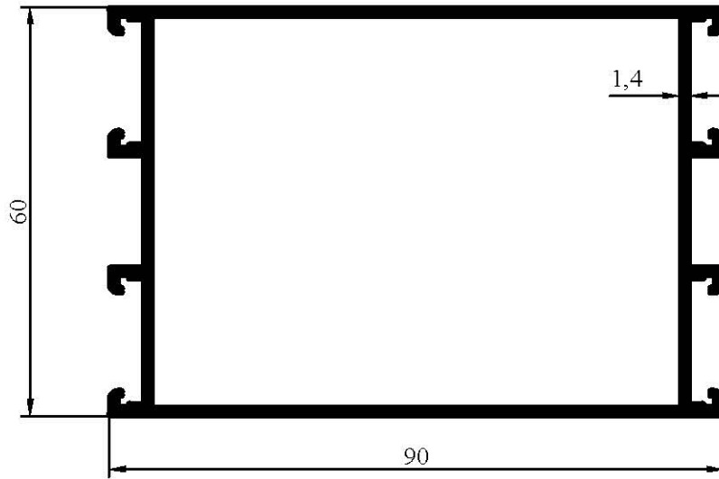
7018 1,298 kg/m
