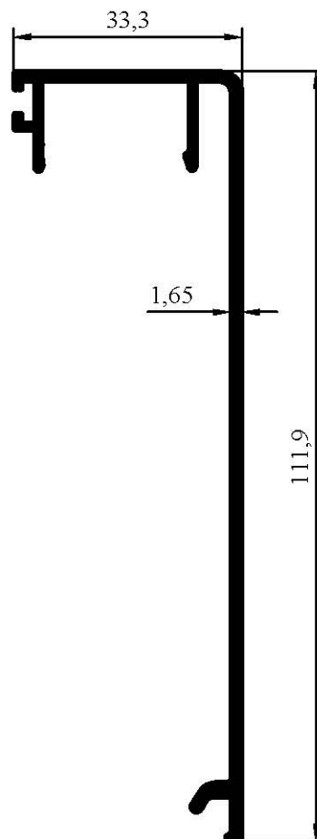
7069 0,763 kg/m
