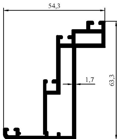
7056 1,062 kg/m
