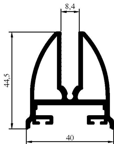
7076 0,949 kg/m
