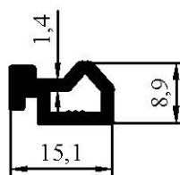
7059 0,172 kg/m
