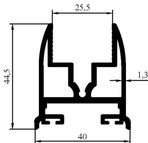
7077 0,981 kg/m
