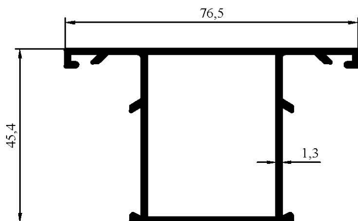
7003 0,828 kg/m
