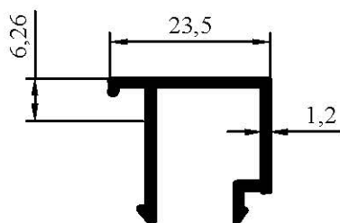
7020 0,228 kg/m
