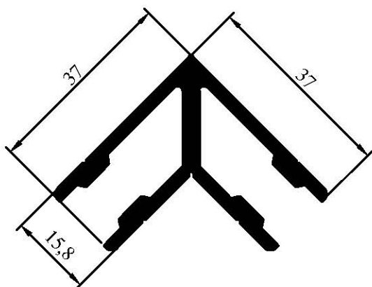
7011 0,913 kg/m
