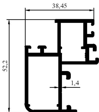
7055 0,881 kg/m
