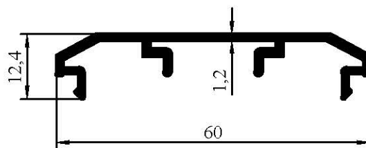
7022 0,369 kg/m
