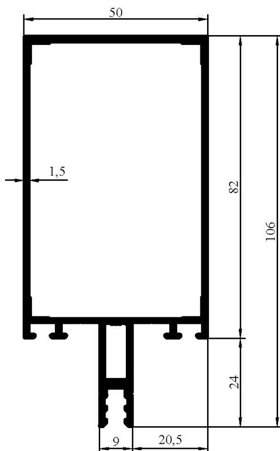
7051 1,444 kg/m
