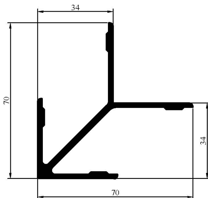
7013 1,171 kg/m
