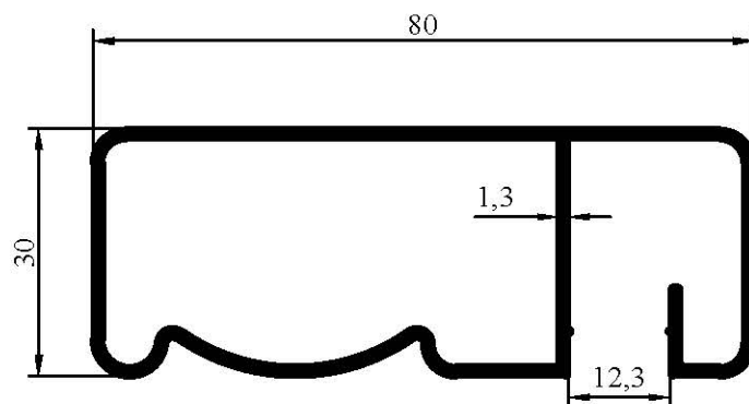
7032 0,830 kg/m
