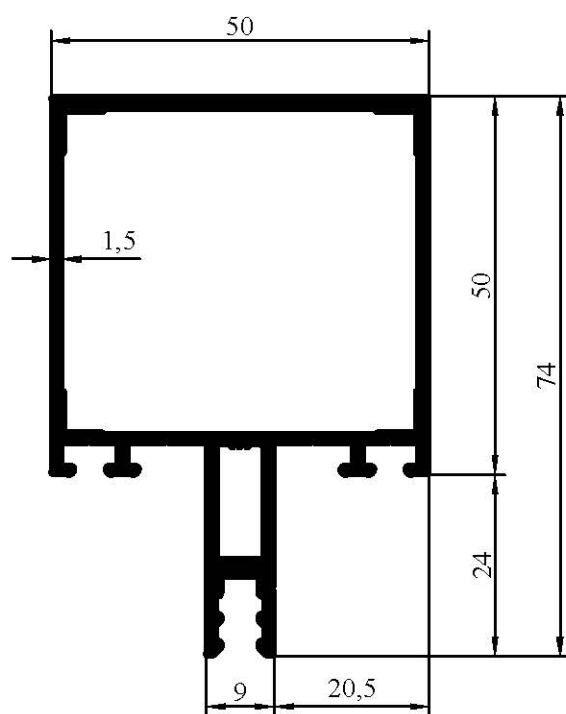
7050 1,184 kg/m
