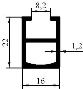
7028 0,265 kg/m
