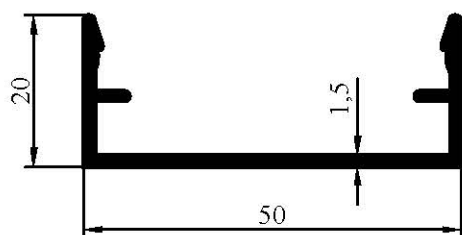
7057 0,403 kg/m
