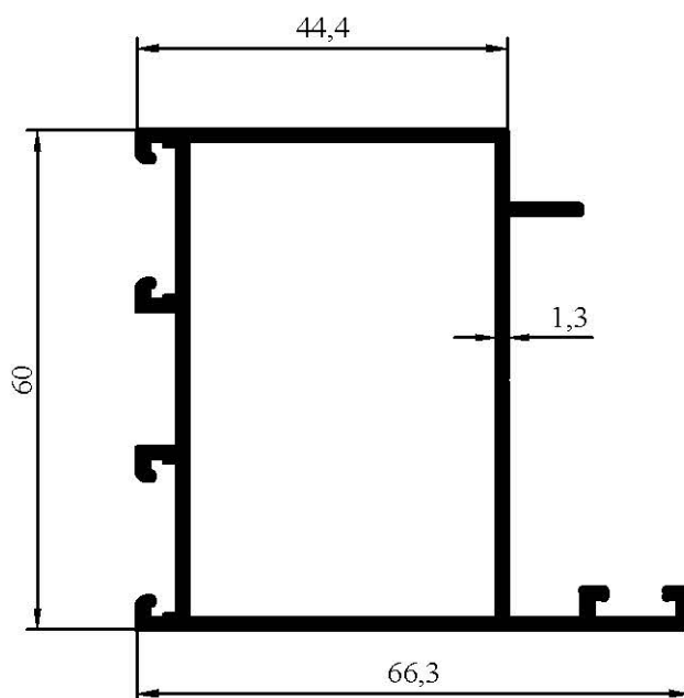
7014 0,946 kg/m
