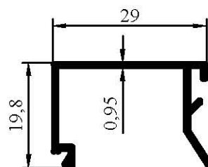
7007 0,203 kg/m
