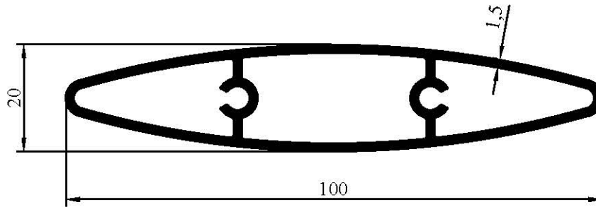
7025 1,028 kg/m
