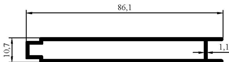
7008 0,563 kg/m
