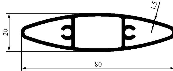
7024 0,902 kg/m
