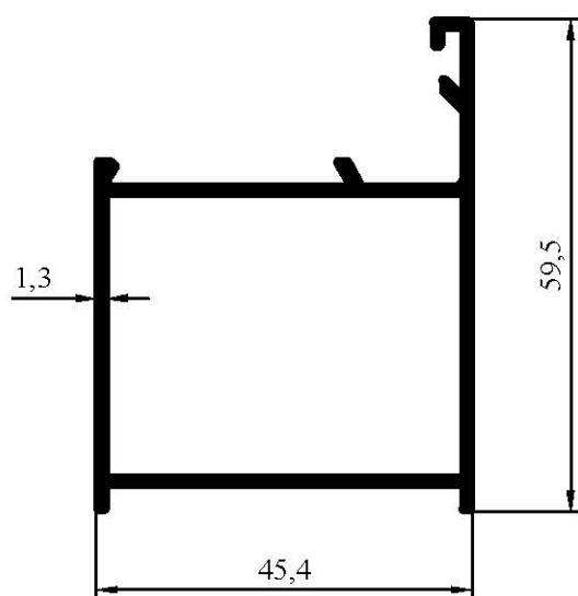
7002 0,714 kg/m
