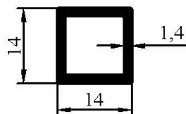
7035 0,191 kg/m
