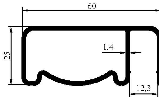
7031 0,678 kg/m
