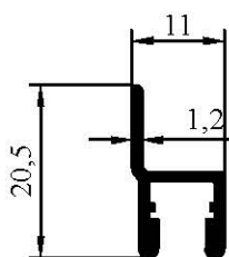
1004 0,144 kg/m
