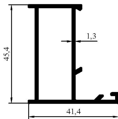
7012 0,587 kg/m
