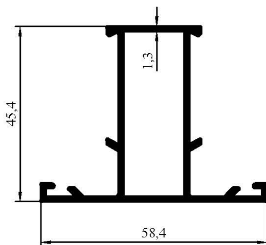
7009 0,700 kg/m
