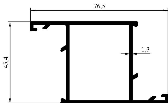
7004 0,828 kg/m
