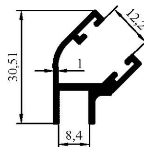
7082 0,282 kg/m
