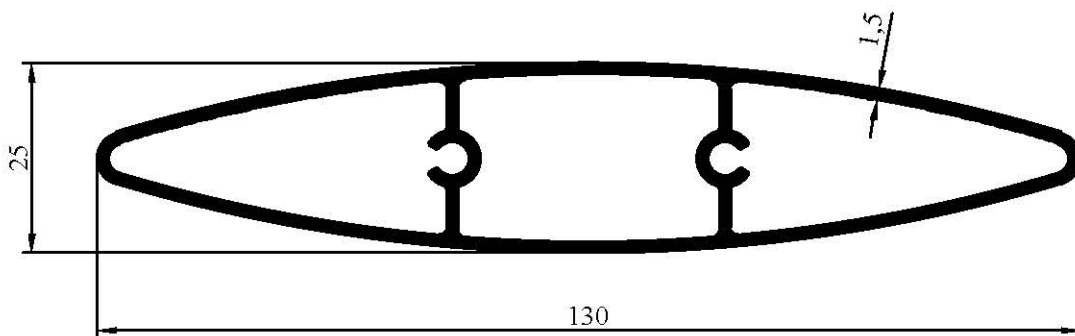
7026 1,323 kg/m
