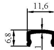
7043 0,060 kg/m
