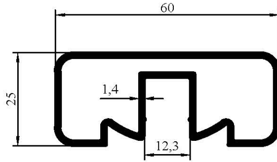
7033 0,768 kg/m
