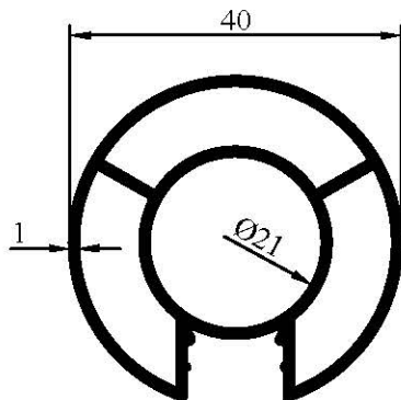
7038 0,582 kg/m
