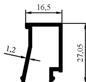
7023 0,244 kg/m
