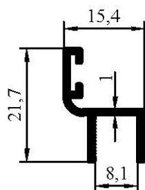
7080 0,152 kg/m
