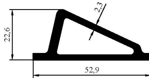
7068 0,794 kg/m
