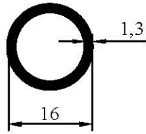
7042 0,163 kg/m
