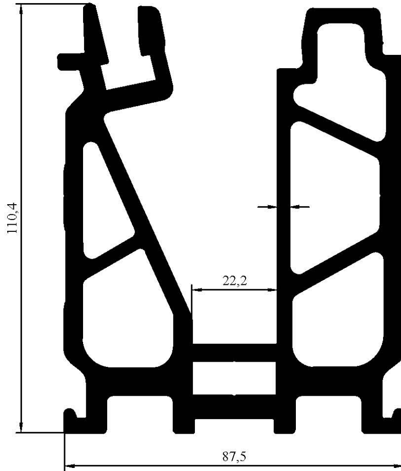
7037 7,610 kg/m
