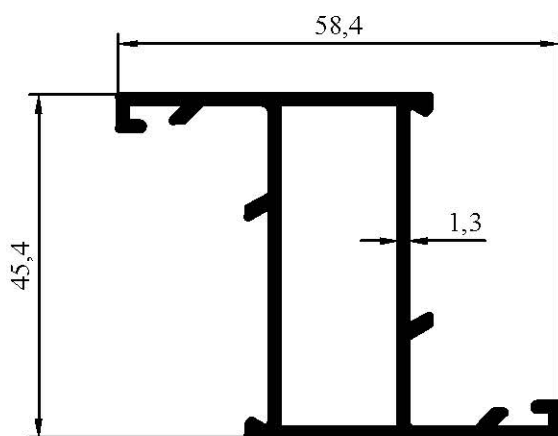
7010 0,700 kg/m
