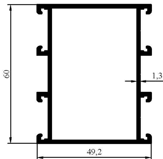
7015 0,913 kg/m
