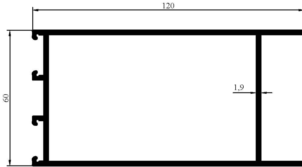
7016 1,891 kg/m
