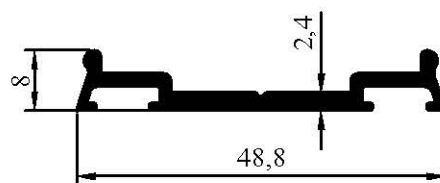
7060 0,353 kg/m
