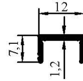
7029 0,064 kg/m
