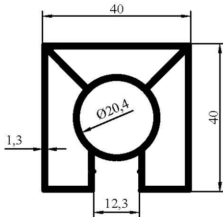
7027 0,914 kg/m
