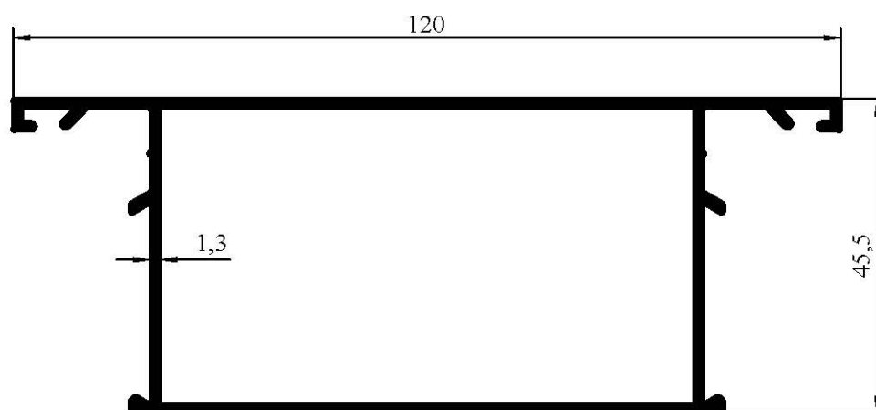
7005 1,130 kg/m
