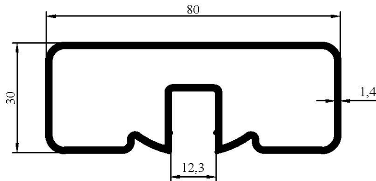
7034 0,938 kg/m
