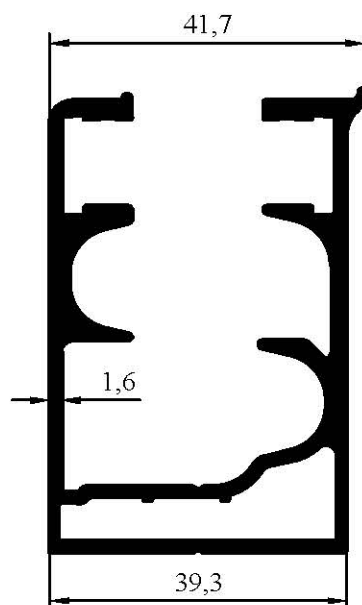
7074 1,252 kg/m
